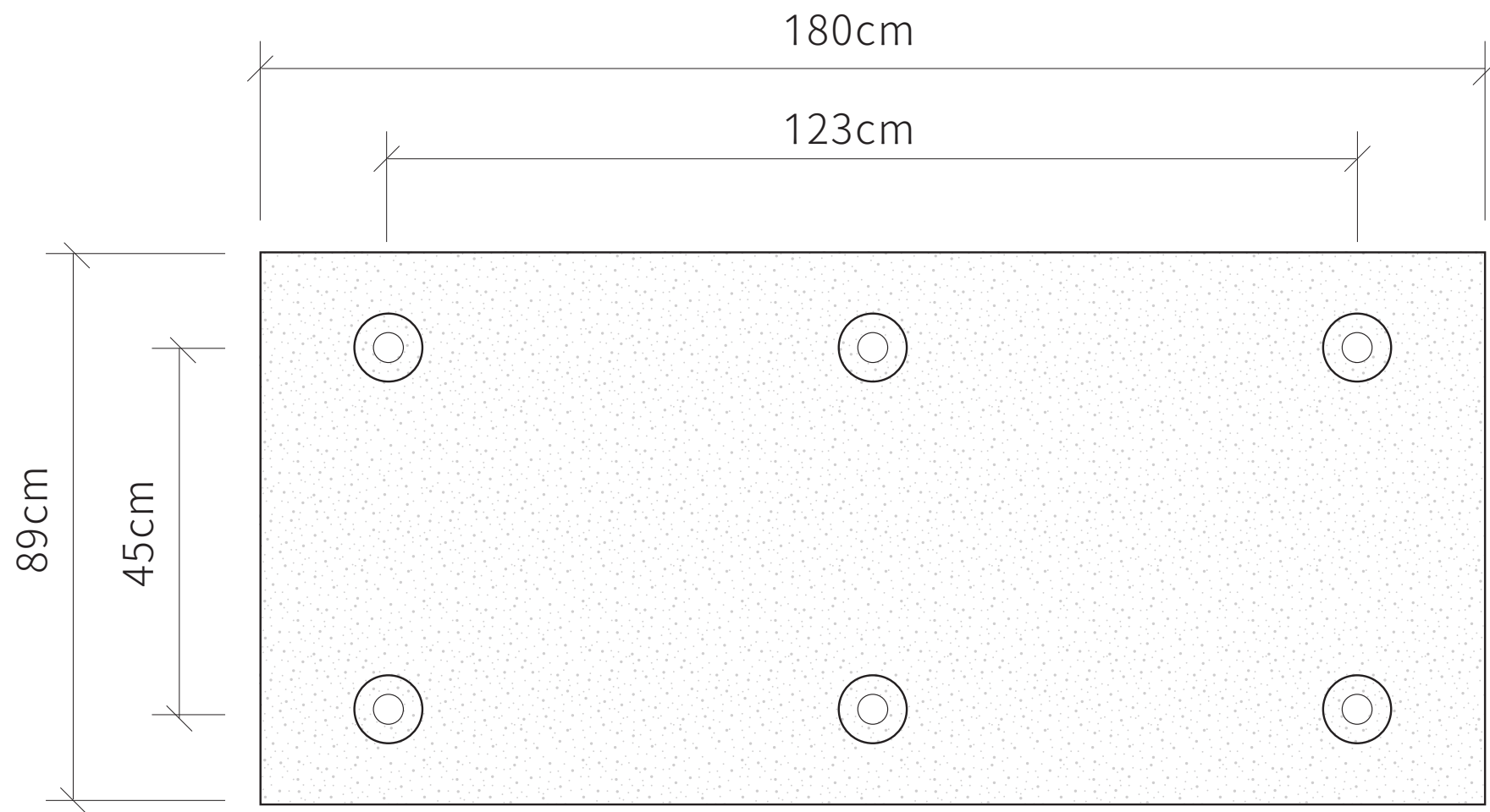
清水模模矩尺寸
