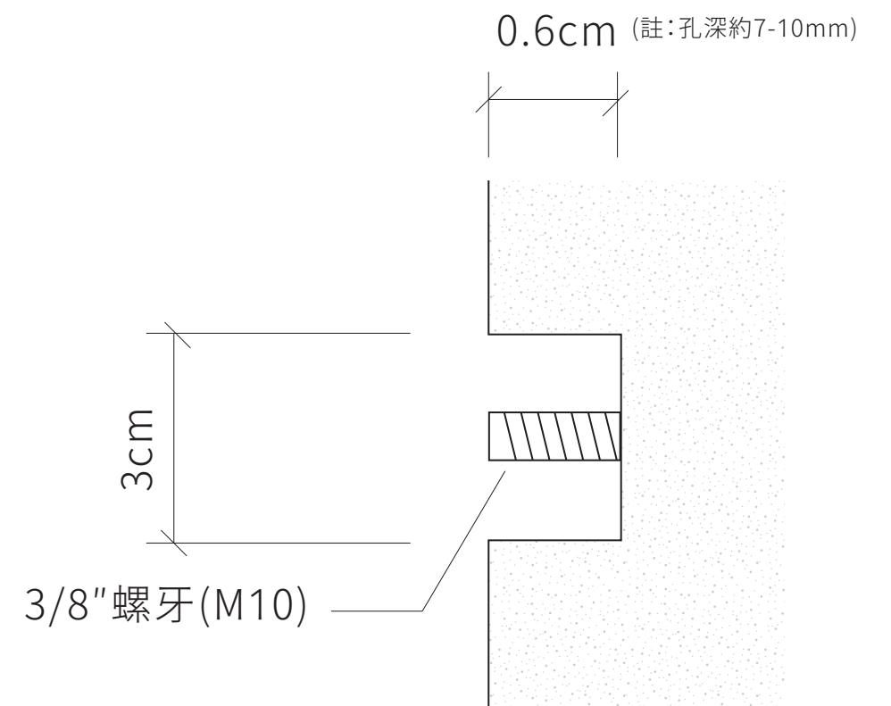
清水模螺栓孔洞剖面
